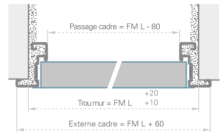
PORTE À UN VANTAIL SECTION HORIZONTALE
