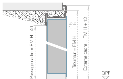
PORTE SANS BATTANT INFÉRIEUR SECTION VERTICALE
