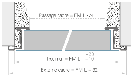
PORTE À UN VANTAIL SECTION HORIZONTALE
