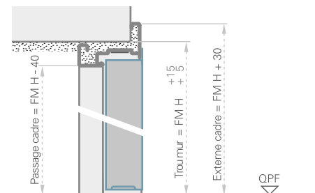
PORTE SANS BATTANT INFÉRIEUR SECTION VERTICALE
