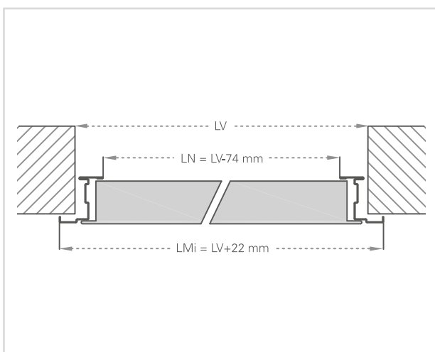
MODÈLE MULTI-USAGE - SECTION HORIZONTALE
