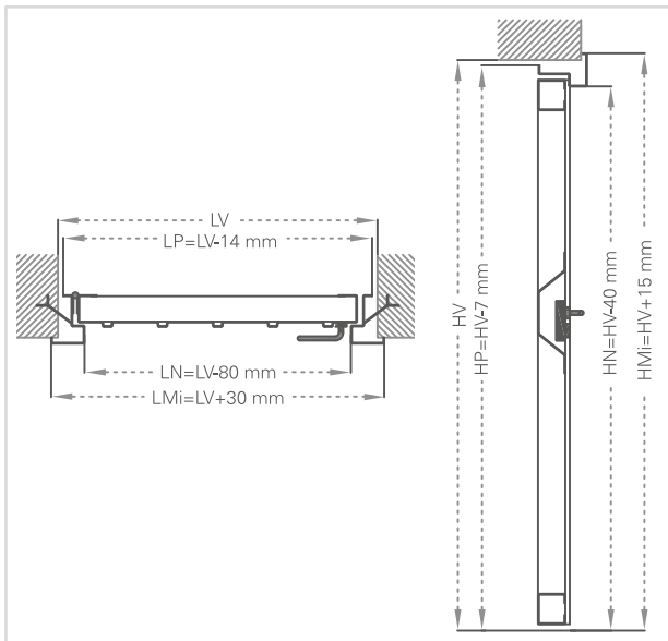
MODÈLE LIGHT - POUSSER
