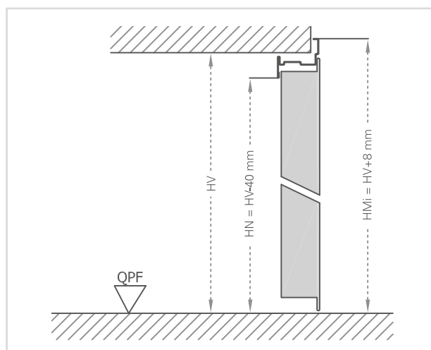
MODÈLE MULTI-USAGE - SECTION VERTICALE
