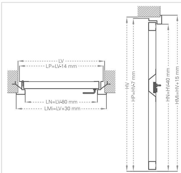
MODÈLE STRONG - POUSSER
