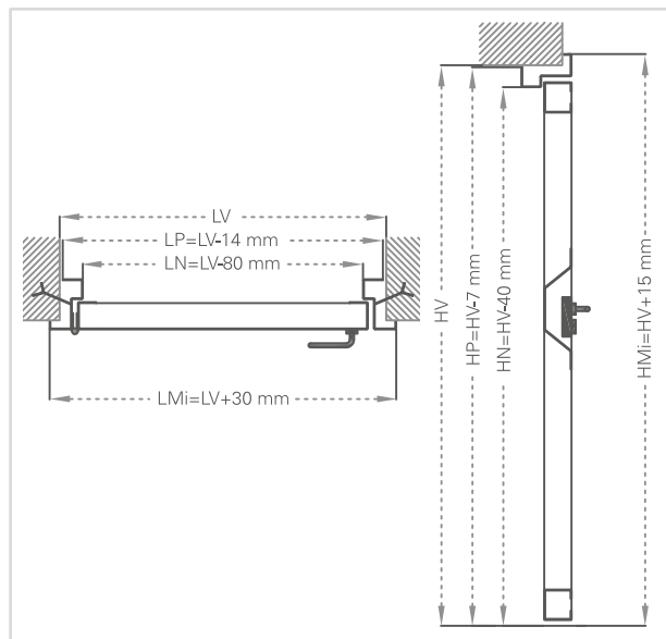
MODÈLE STRONG - TIRER
