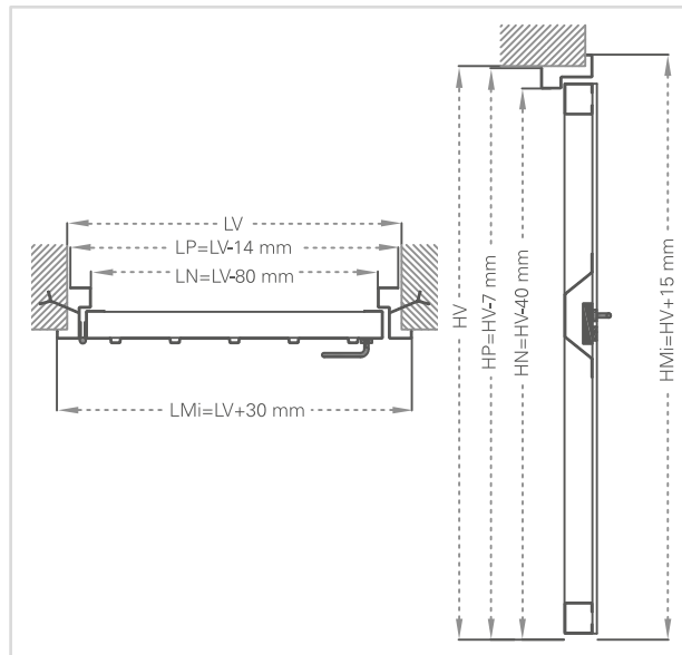
MODÈLE LIGHT - TIRER
