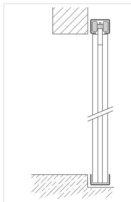
MONTAGE À L'EXTÉRIEUR DE L'OUVERTURE DE LA PAROI
