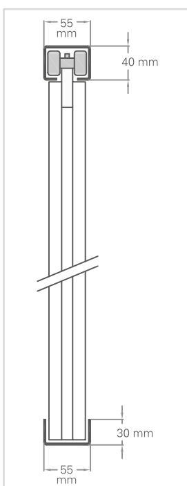
SECTION LATÉRALE
